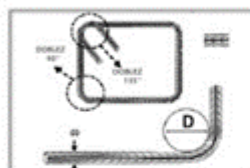
3_Doblado Varillas
