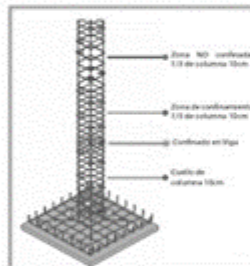
5_Armado Columna
