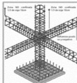
6_Armado Viga
